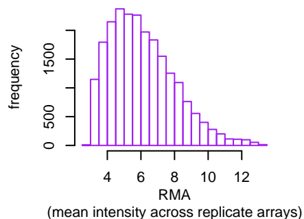
f) Histogram
