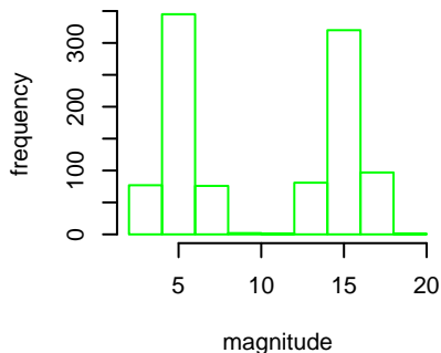
e) Histogram
