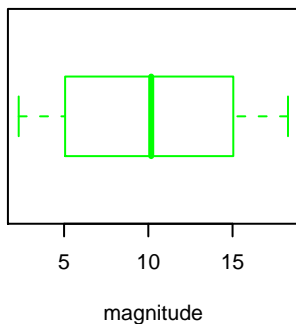
b) Boxplot
