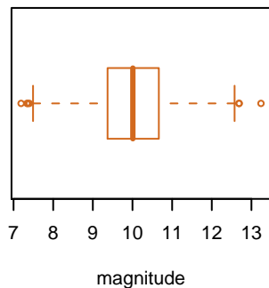
a) Boxplot
